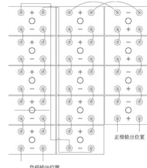
图2 HKFM-600 蓄电池组连接示意图 (一)
