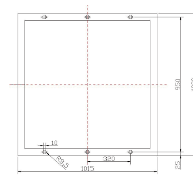
图4 HKFM-600 蓄电池安装架底座孔位图
